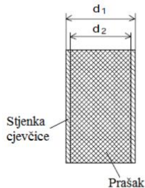
Slika 2.10 Praškom punjena žica[4]
