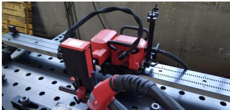
Slika 2.8 Automat za MIG/MAG zavarivanje [1]
