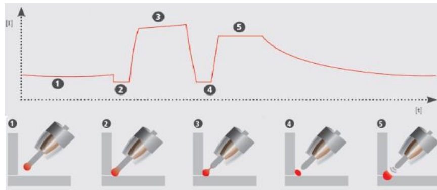
Slika 2.5 LSC prijenos metala kratkim spojem [1]
